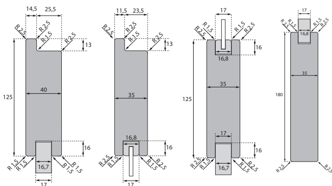
Riegel seitlich
